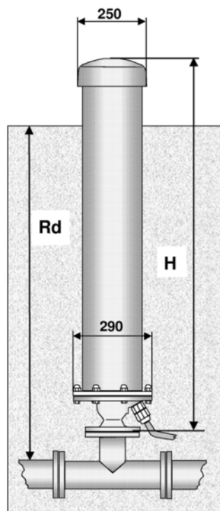
Надземная установка
